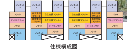
住棟構成図
