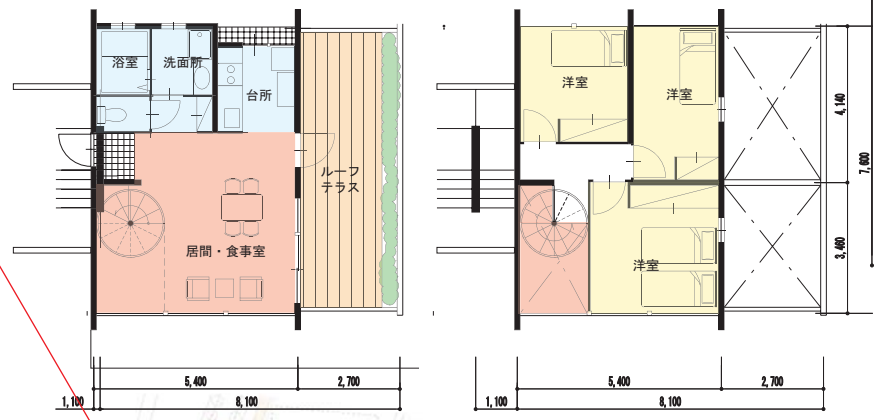
メゾネット5 住戸平面図 S=1/100
